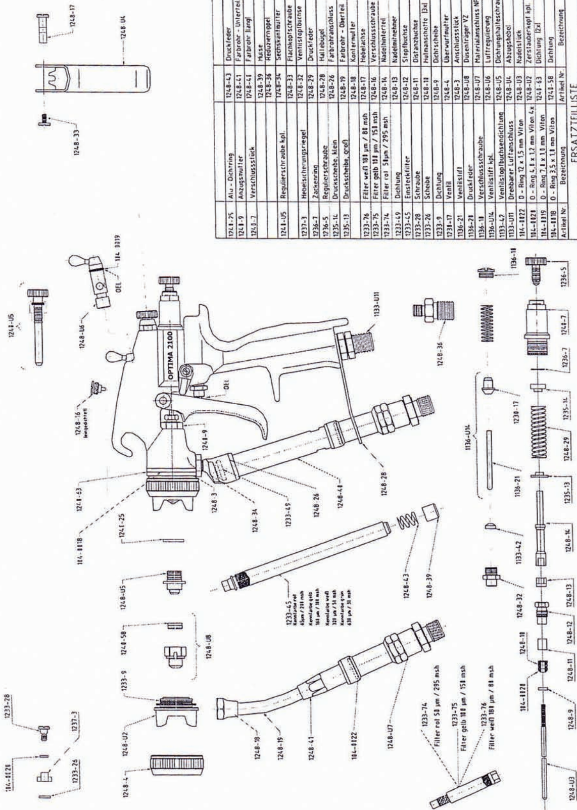
Abbildung 4: Explosionszeichnung der Optima 2100
